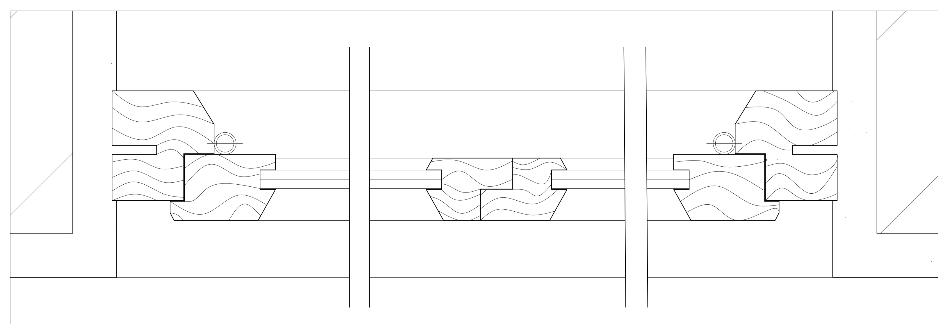
Pormenor Caxilho_esc:1/1
