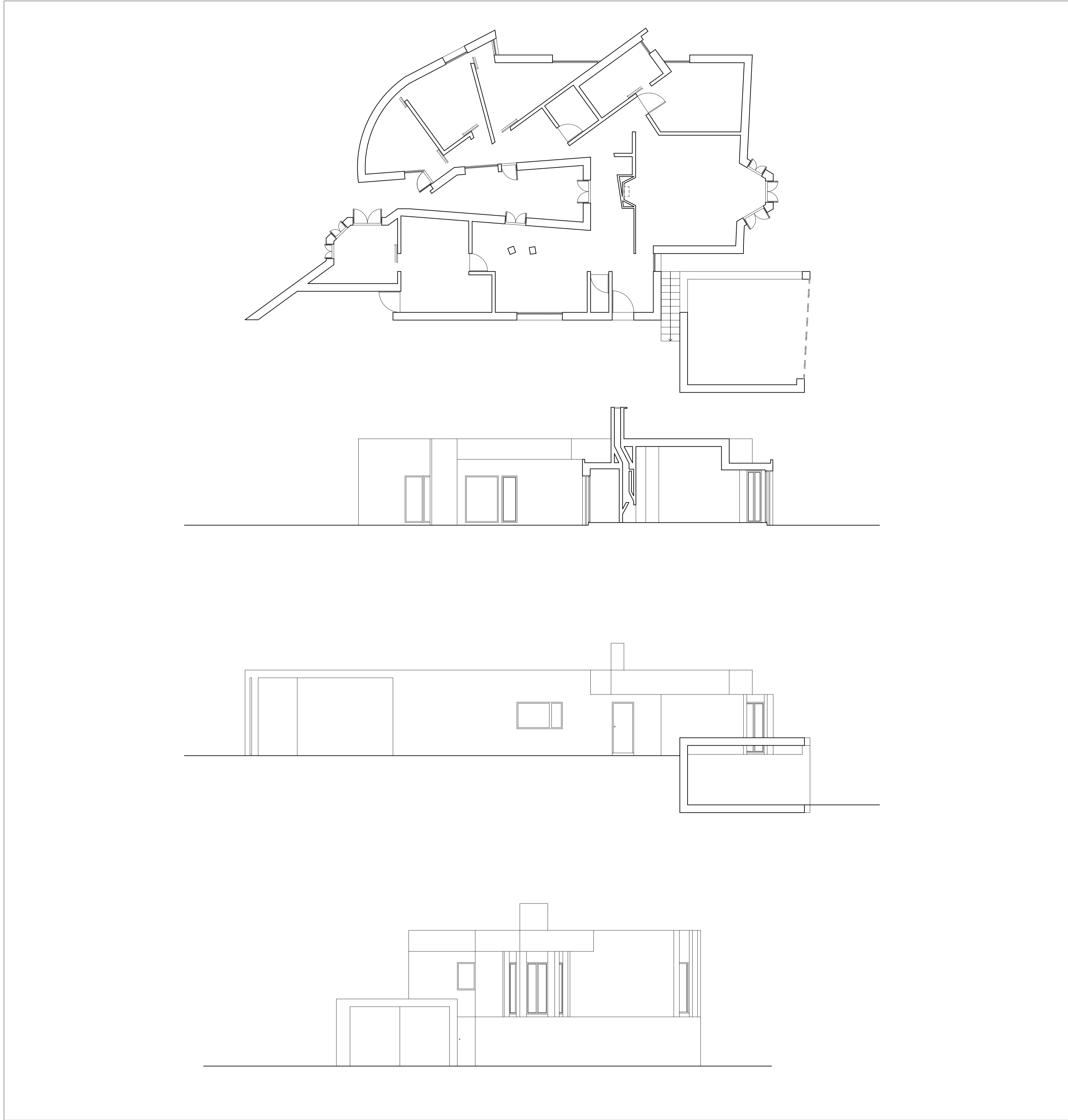
Planta, Corte e alçados_esc:1/100
