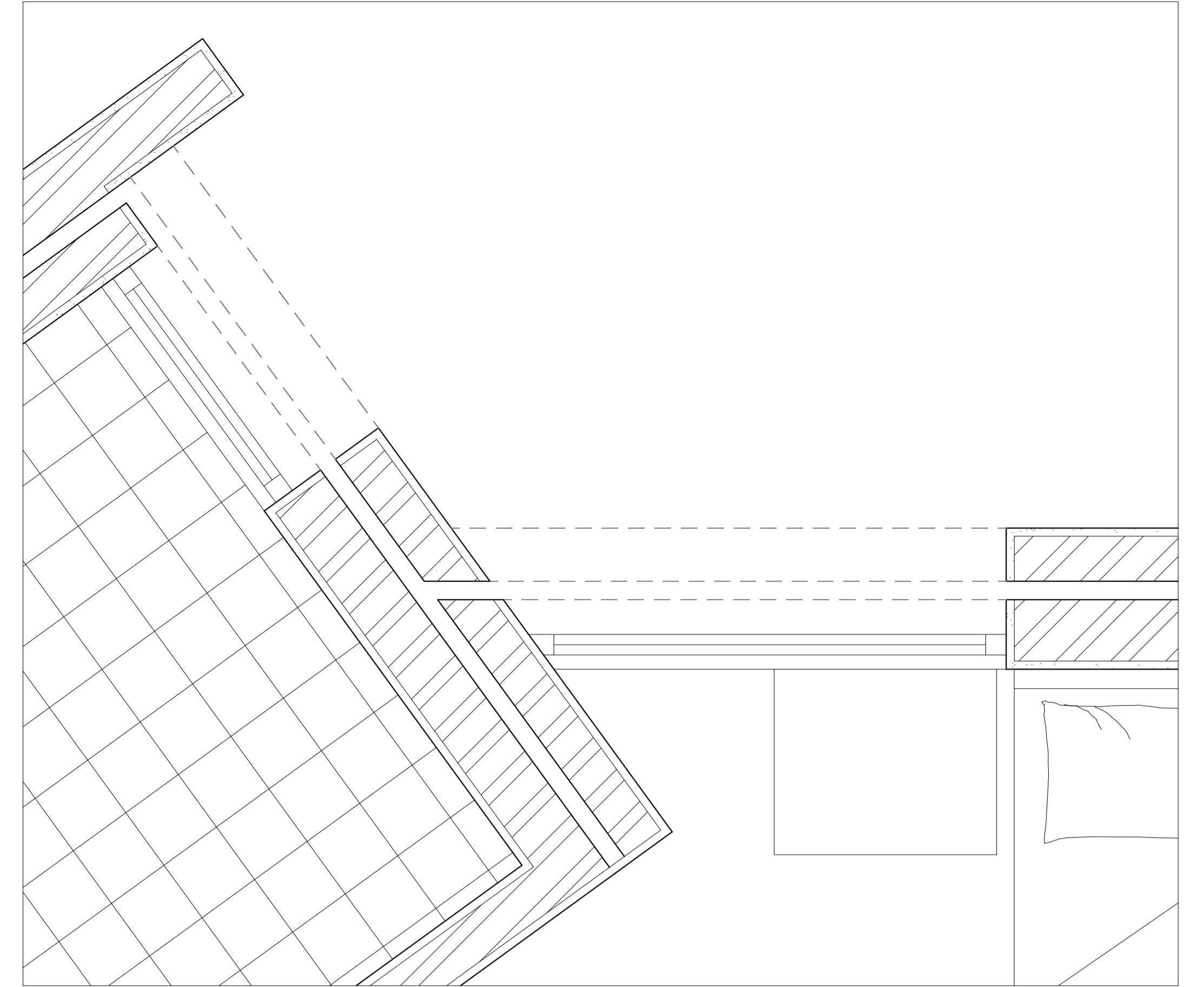
Pormenor Planta_esc:1/10
